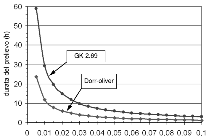
Figura 2 - Durata del prelievo in funzione della concentrazione di SLC aerodispersa per 30 µg di quarzo sul filtro: la curva inferiore si riferisce all'uso del superiore GK 2.69 a 4,2 L/min mentre l'altra si riferisce al Dorr-Oliver a 1,7 L/min
