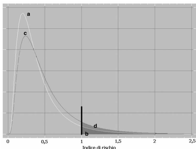
Figura B2 - Curva limite e curva per una situazione di superamento del limite
